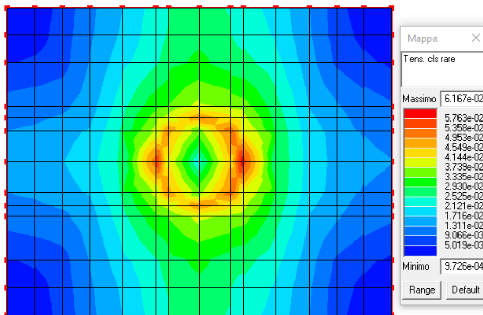
Figura 24: Verifica tensioni rare nel cls.
