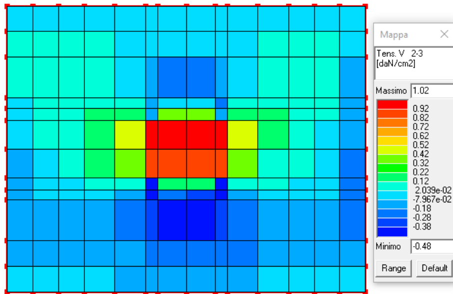
Figura 20: Tensioni di taglio 2-3 in daN/cm².
