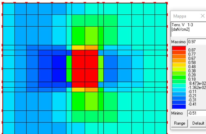
Figura 19: Tensioni di taglio 1-3 in daN/cm 2 .
