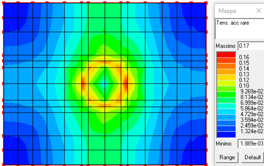
Figura 25: Verifica tensioni rare nell'acciaio.
