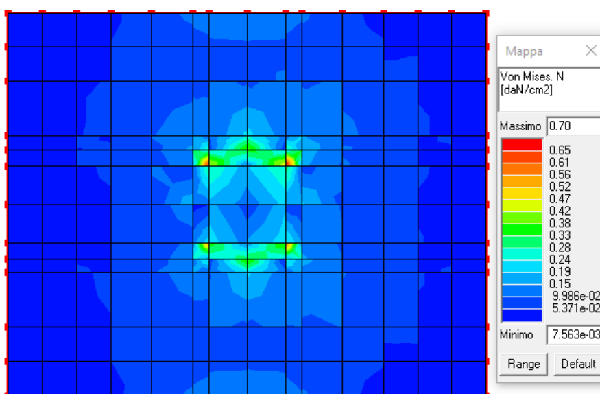
Figura 17: Tensioni di membrana (N) tramite formulazione di Von Mises.
