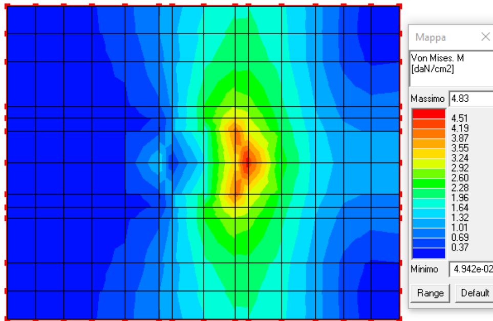
Figura 18: Tensioni di flessione (M) tramite formulazione di Von Mises.
