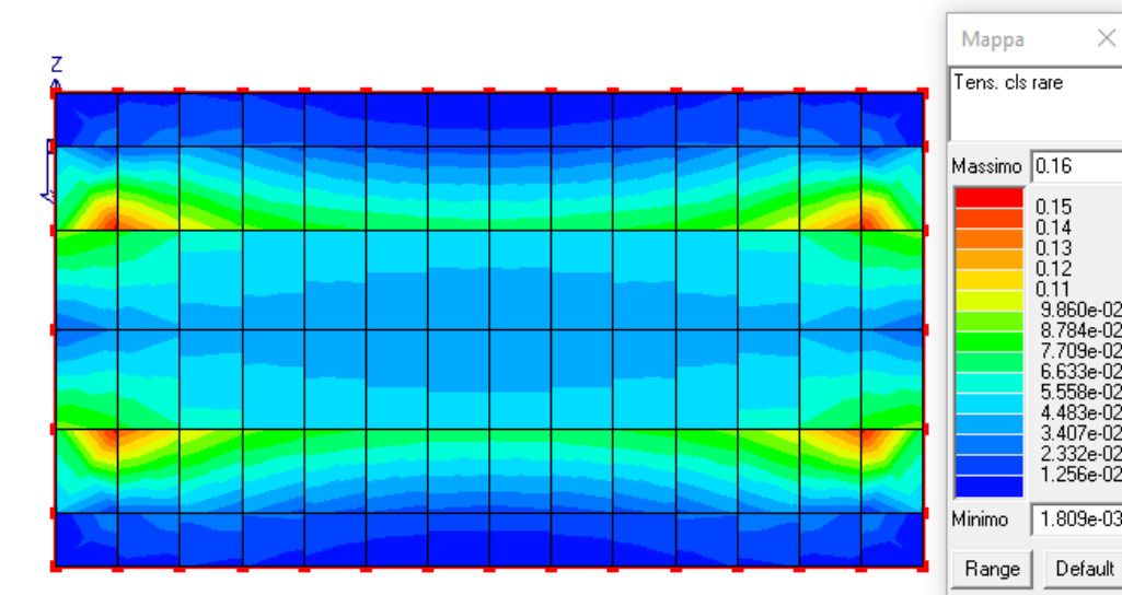
Figura 23: Verifica tensioni rare nel cls.
