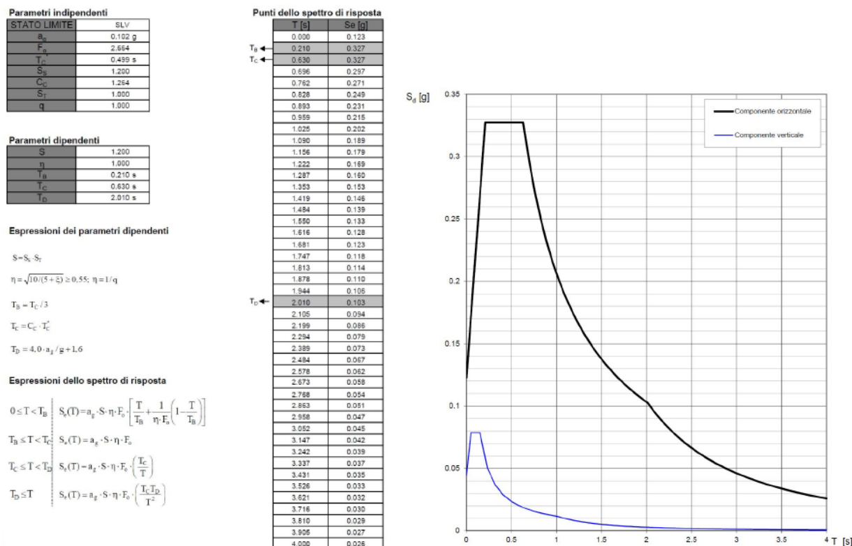
Figura 13: Parametri spettro di risposta SLV.
