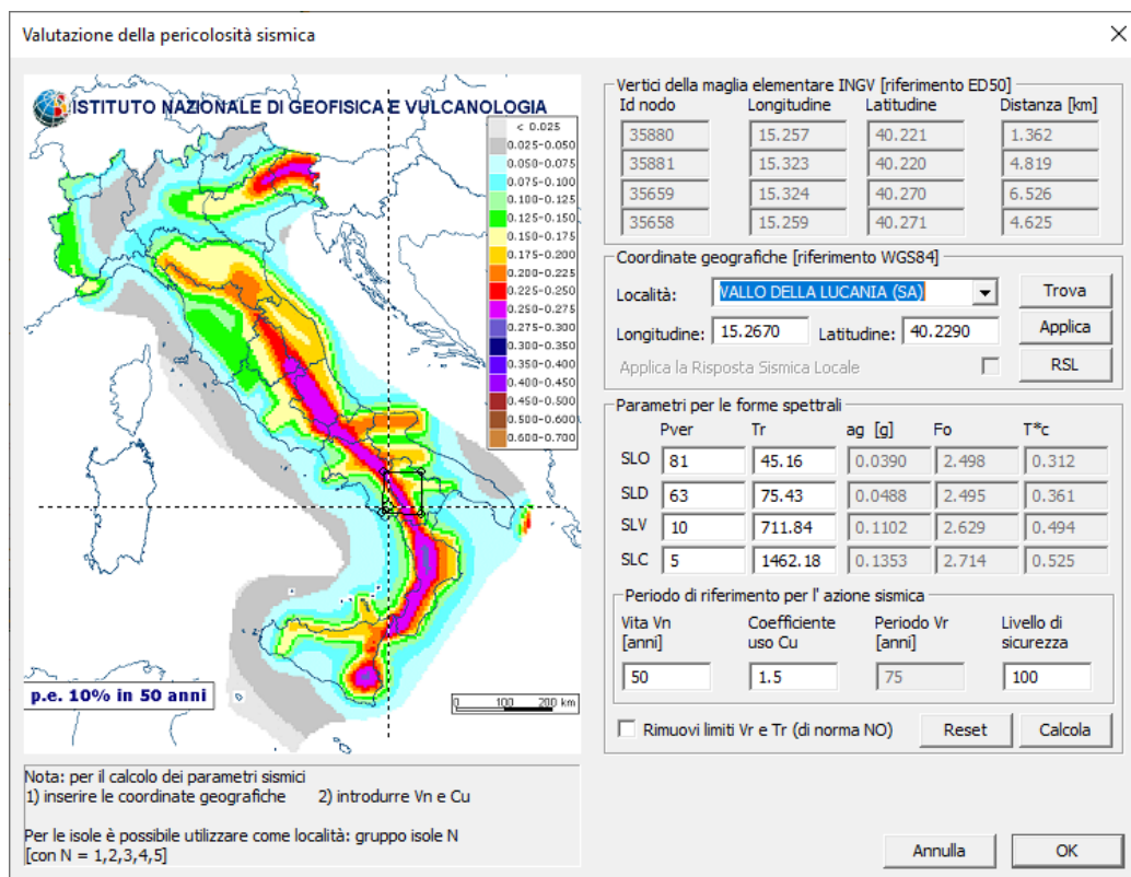
Figura 4: Valutazione della pericolosità sismica.
