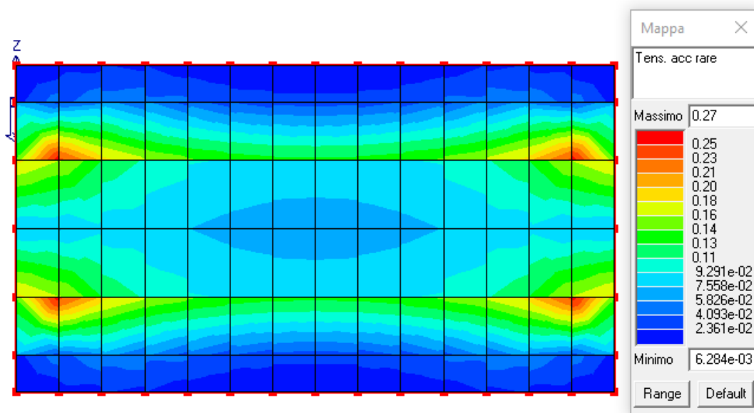
Figura 24: Verifica tensioni rare nell'acciaio.
